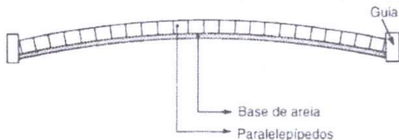
Figura 6.1 Seção típica para ruas
